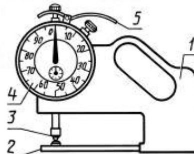
1 — корпус; 2 — неподвижный стержень; 3 — измерительный наконечник; 4 — отсчетное устройство; 5 — арретир
